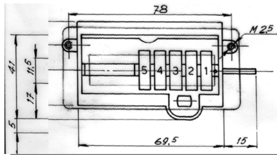
Dimensioni d'ingombro
